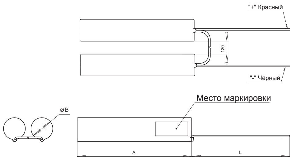
Габаритный чертеж АКБ
