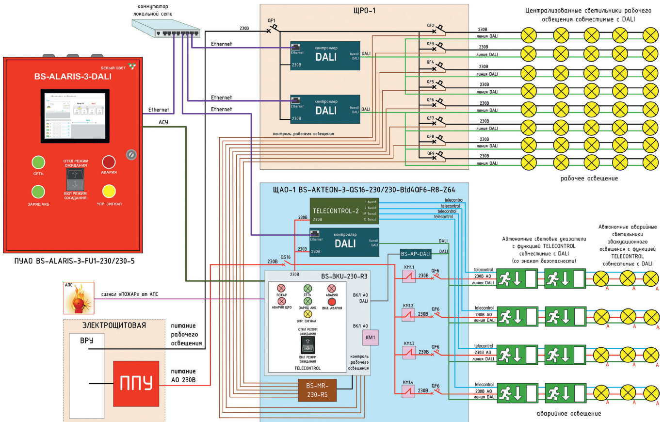
Автономная система аварийного освещения ZARIUS DALI (однофазная, 230В) с функцией TELECONTROL
