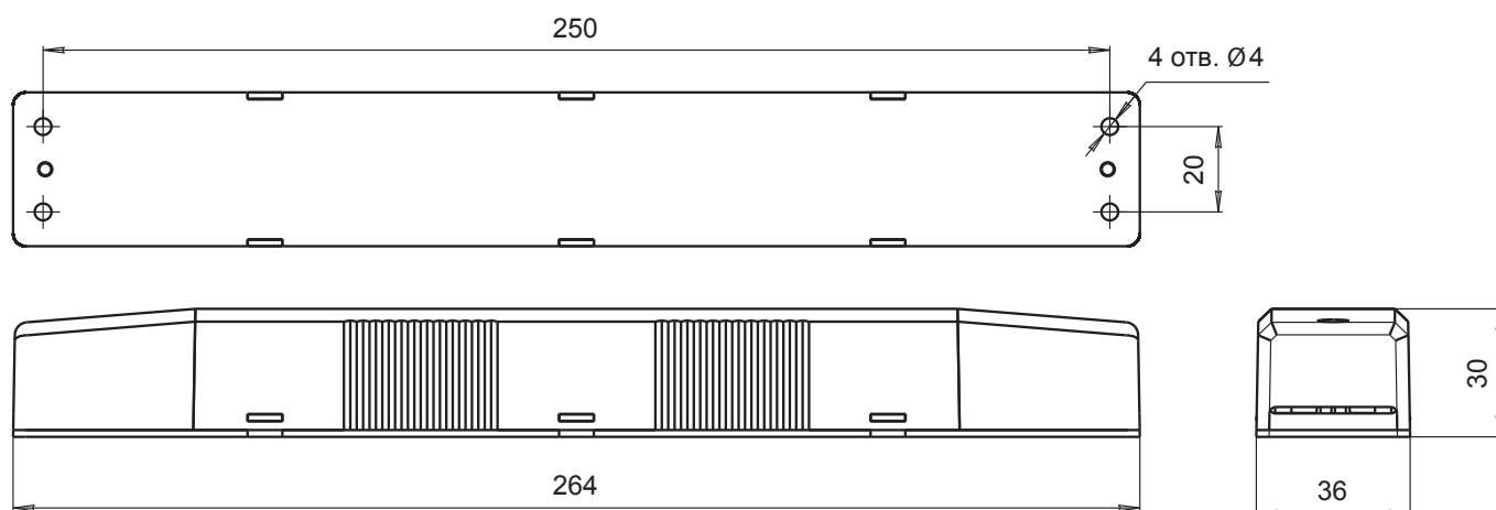
Блоки аварийного питания BS-STABILAR2-B1/B2-LED
